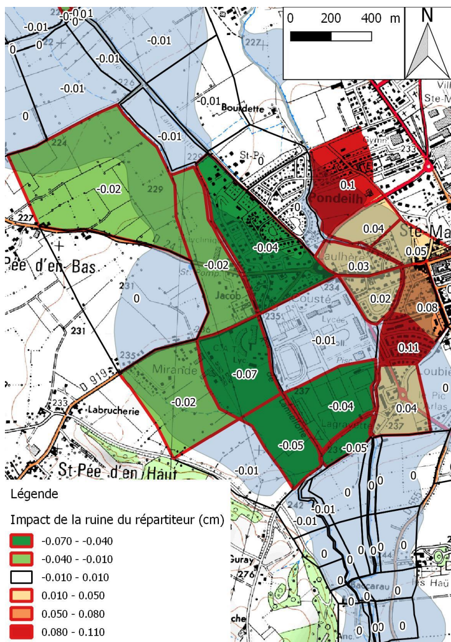
Fig. 67. Impact de la ruine du partiteur sur les niveaux maximum aux casiers à Oloron
