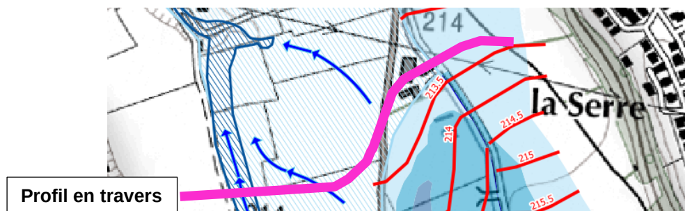
Fig. 54. Profil en travers du lit majeur de la Mielle à l'isocote 213.5
