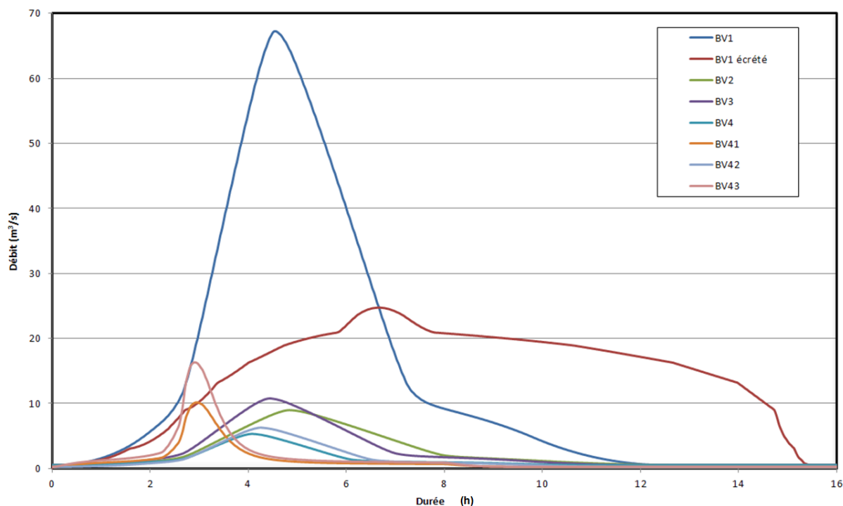
Fig. 39. Débits générés sur les Mielles par la pluie centennale de référence
