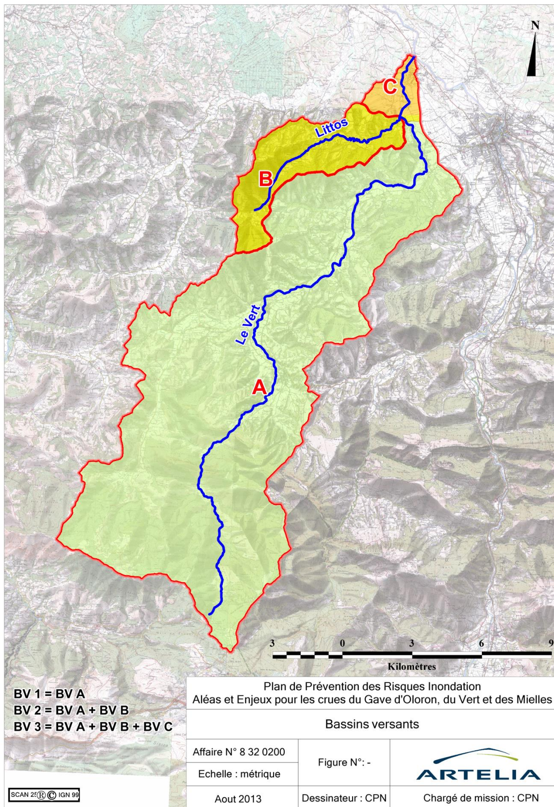
Fig. 37. Bassins versants
