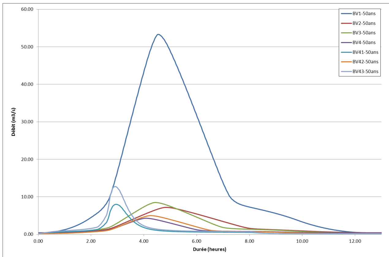
Fig. 42. Hydrogrammes des sous bassins versants pour T = 50 ans
